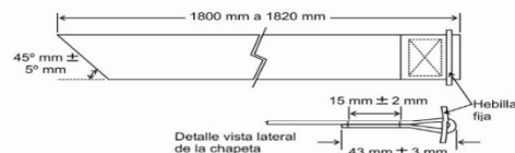
Figura 1. Correa y accesorios del portafusil ensablado
